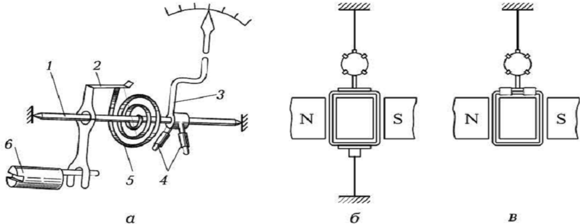
Рис. 3.1. Способы задания противодействующего момента:
