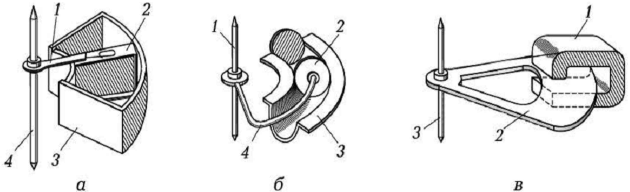
Рис. 3.3. Типы успокоителей:
