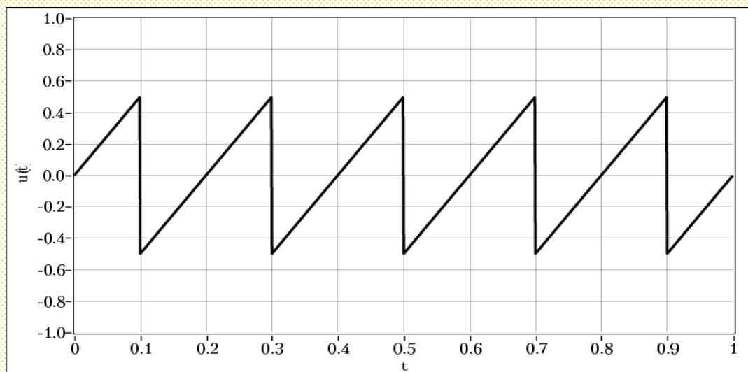
пилообразный сигнал
