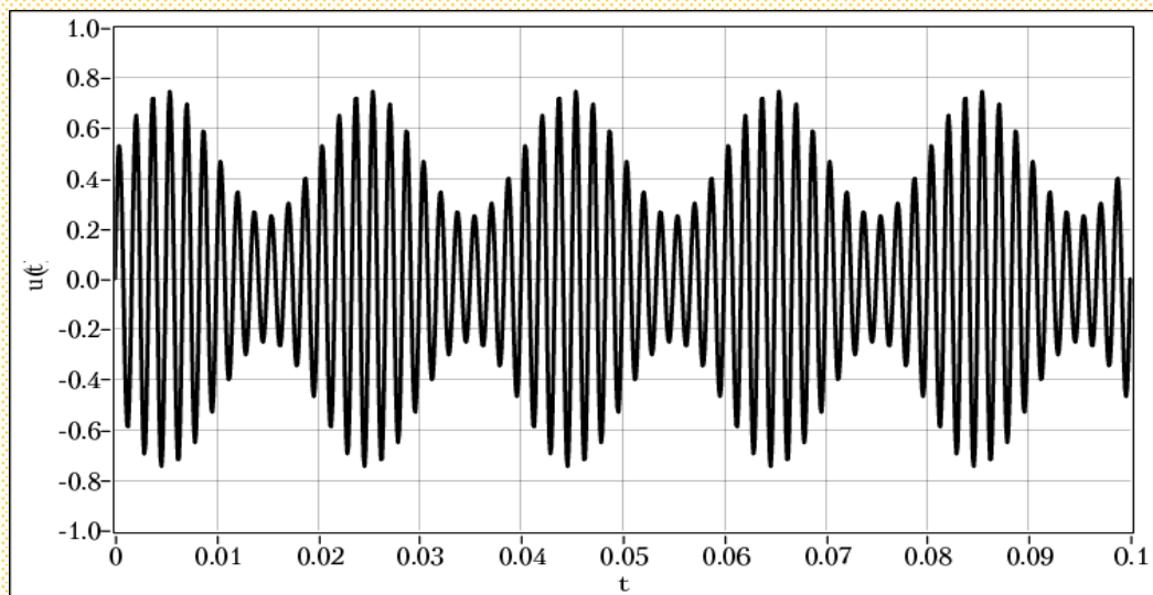
Амплитудная (АМ)
