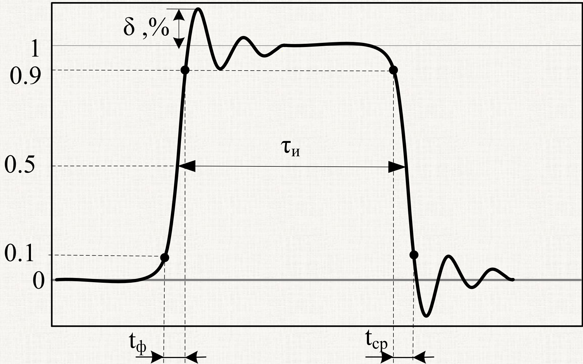
Вид реального импульса, близкого к прямоугольному
