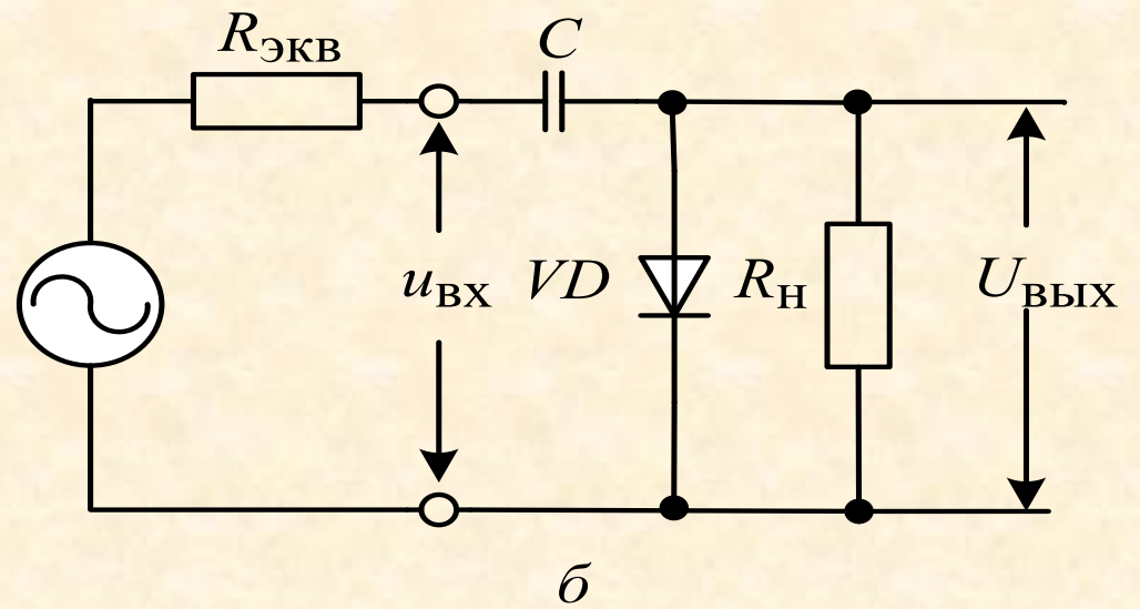
Амплитудный детектор: а – с открытым входом; б – с закрытым входом
