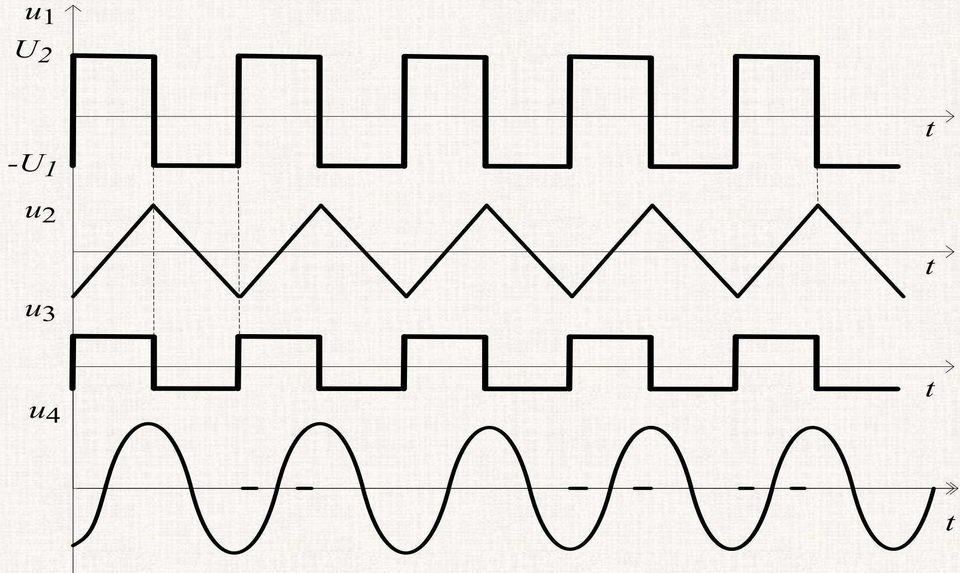
Диаграммы напряжений функционального генератора
