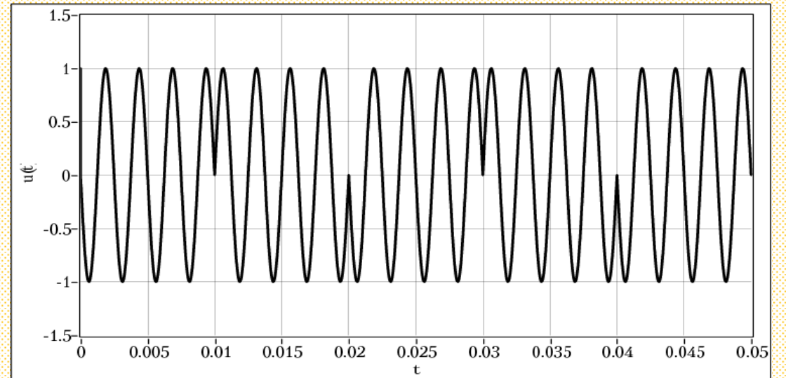
Фазоимпульсная манипуляция
