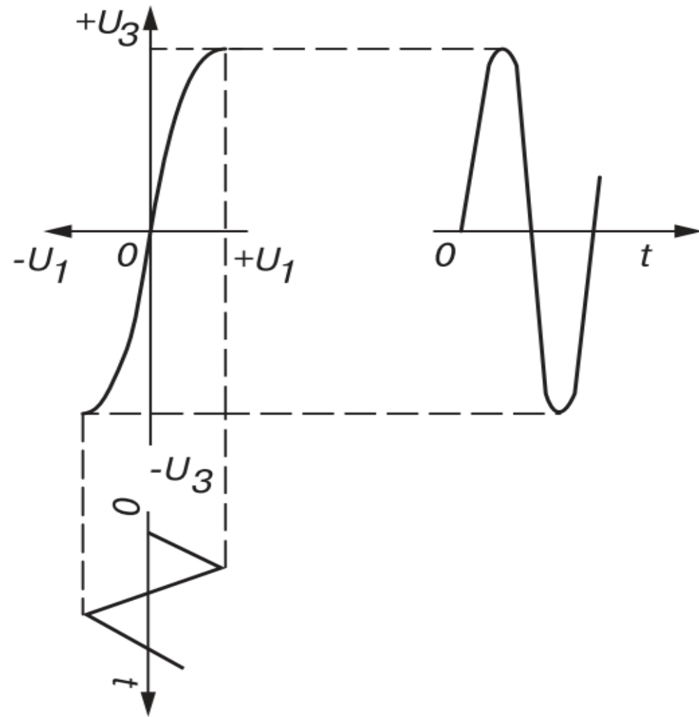
Диаграммы напряжений преобразователя «треугольник - синус»
