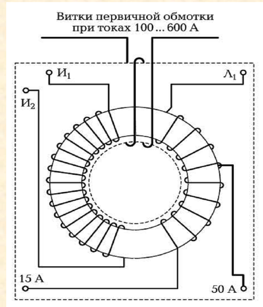
Конструкция тороидального трансформатора тока
