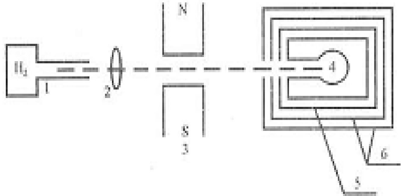
Рис. 2.4. Структурная схема водородного генератора: 1 – баллон с водородом; 2 – коллиматор; 3 – осевой магнит; 4 – накопительная ячейка; 5 – резонатор; 6 – многослойный экран
