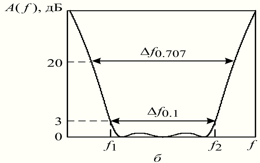
Типичные АЧХ полосно-пропускающего фильтра
