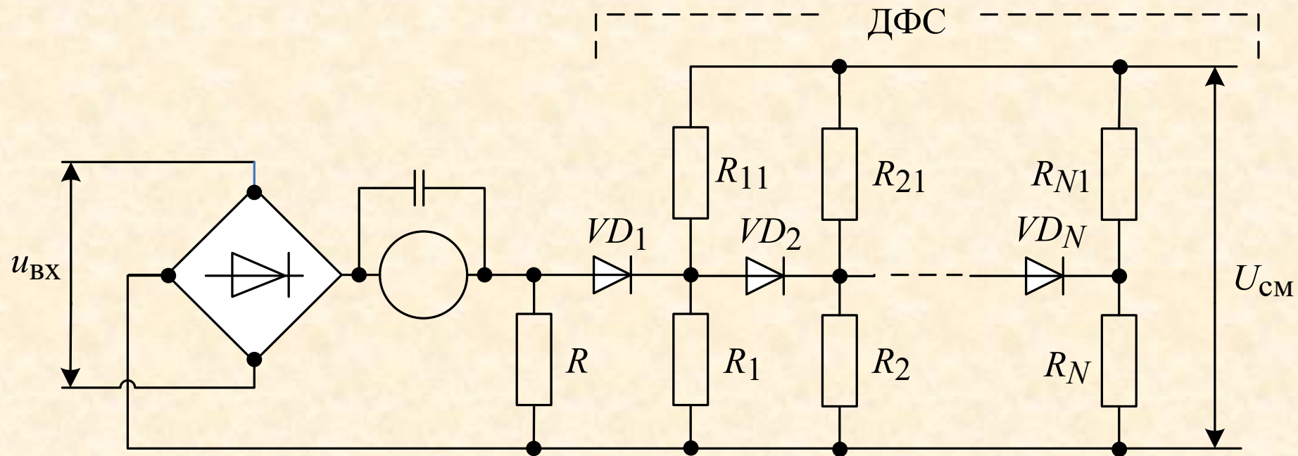
Схема детектора среднеквадратичных значений с ДФС
