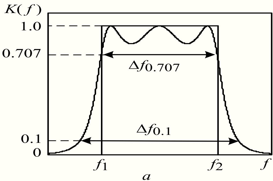
Типичные АЧХ полосно-пропускающего фильтра
