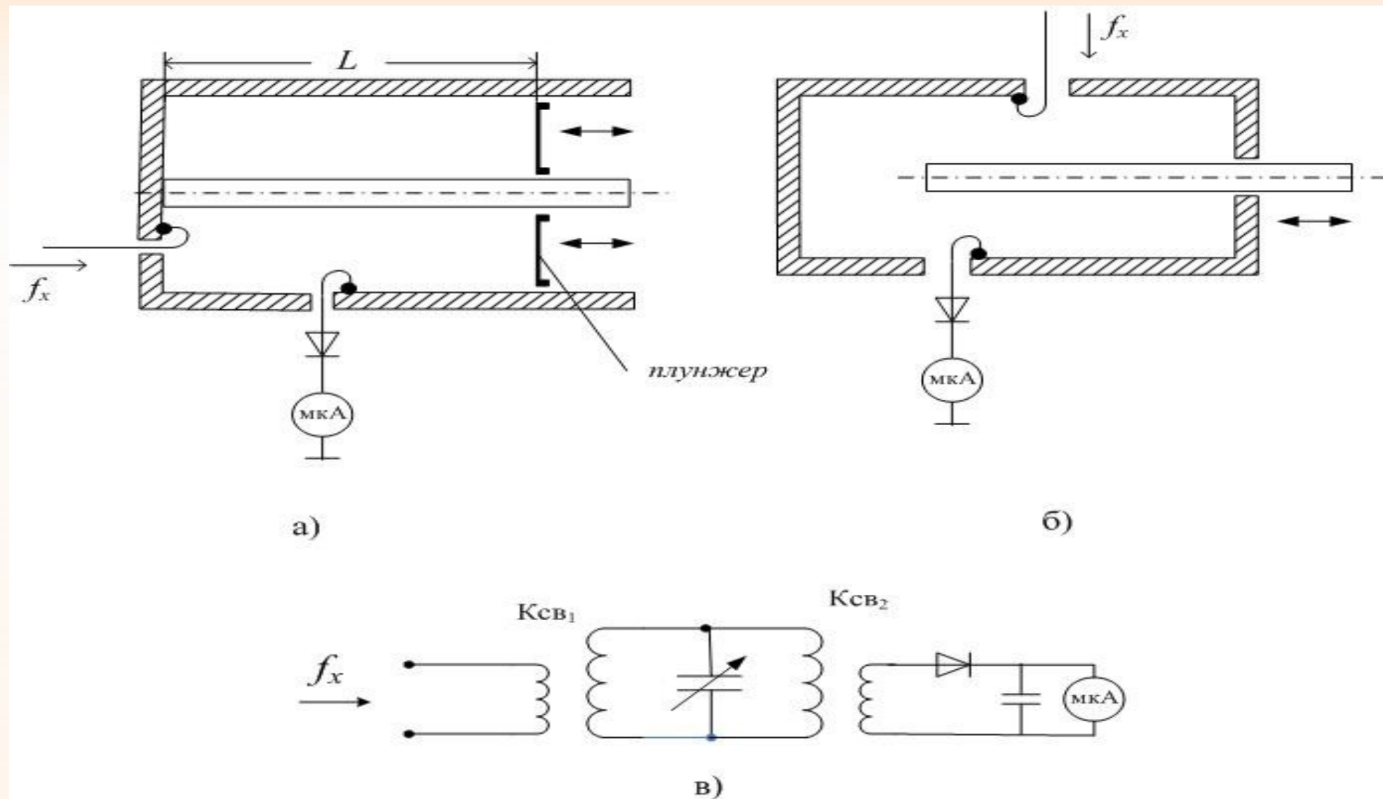
Коаксиальные резонансные частотомеры: а- полуволновый; б – четвертьволновый; в - проходная схема частотомера
