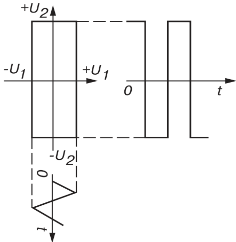
Диаграммы напряжений релейного преобразователя «треугольник- меандр»
