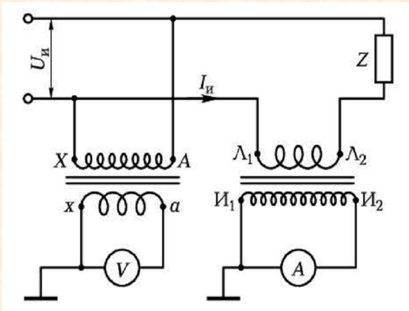
Трансформаторы напряжения и тока
