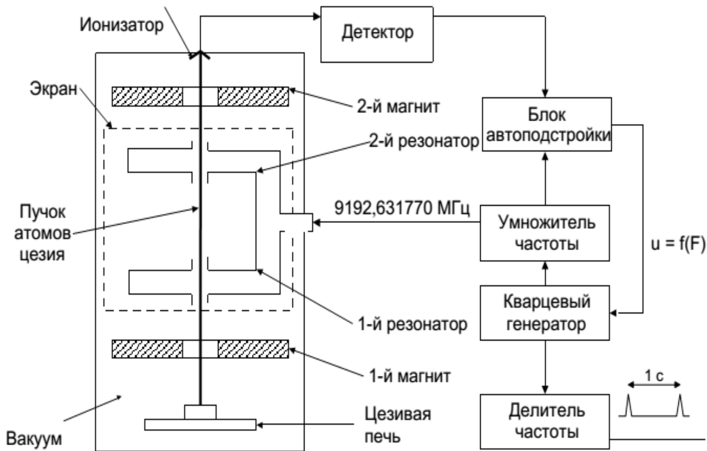
Рисунок 3. Государственный первичный эталон единицы времени и частоты
